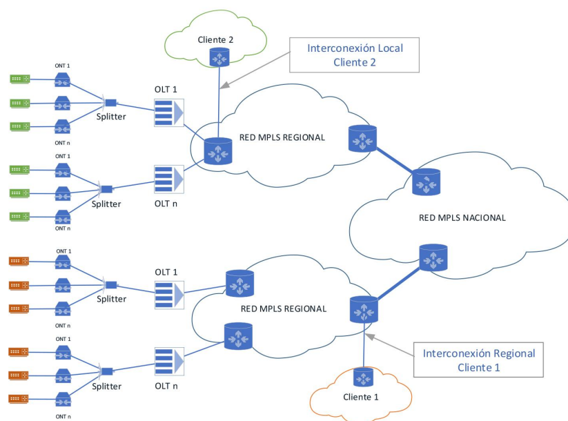
Figura 6 - Interconexión - Conectividad regional
