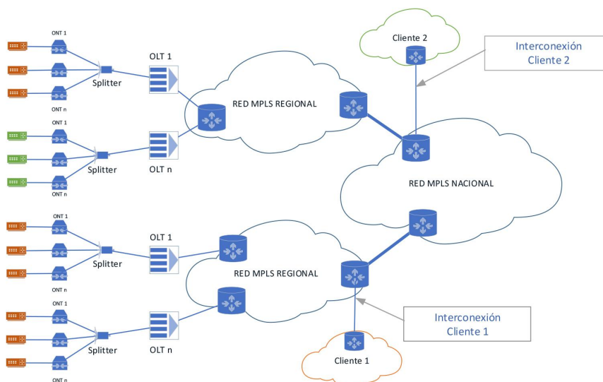
Figura 7 - Interconexión - Transporte de tráfico
