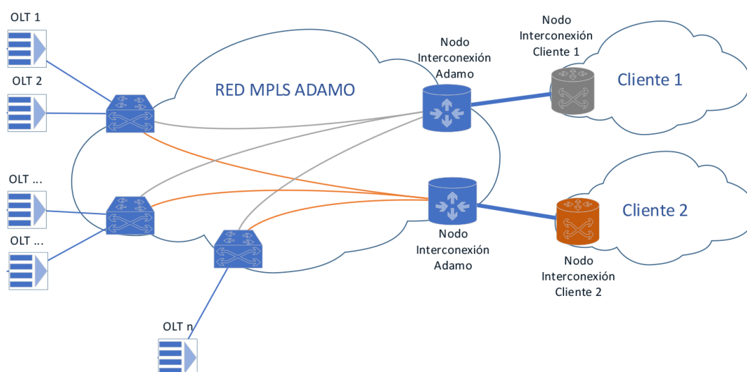
Figura 10 - Servicio OLT Rental
