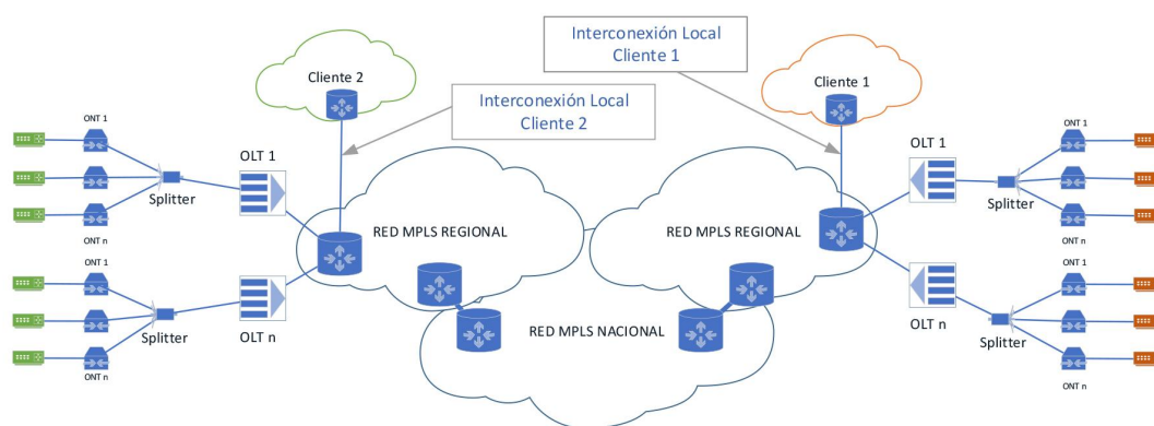
Figura 5 - Interconexión - Conectividad local
