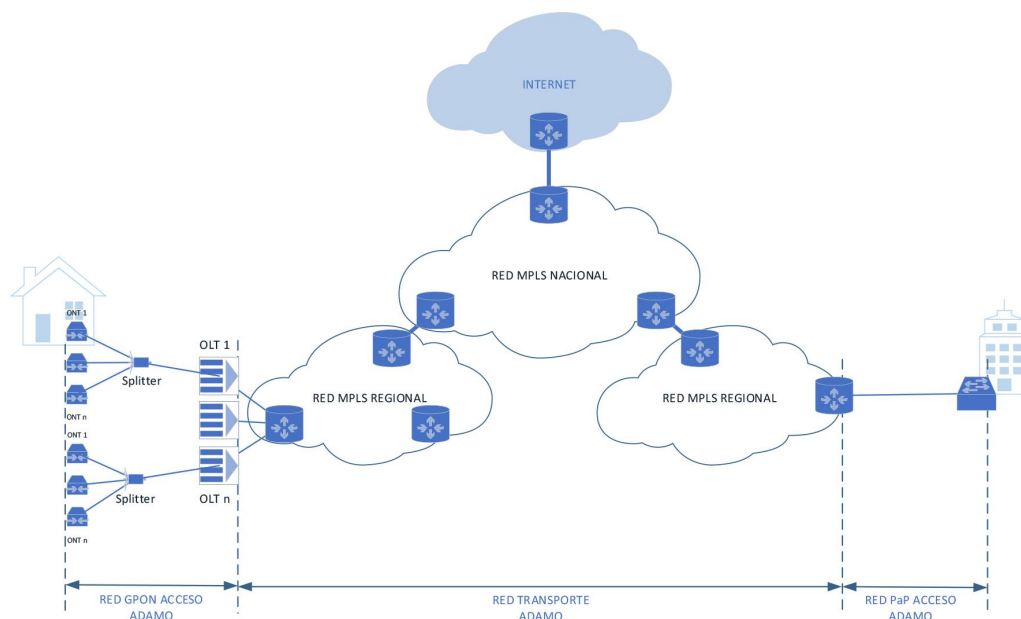
Figura 9 - Servicio Internet Marca Blanca
