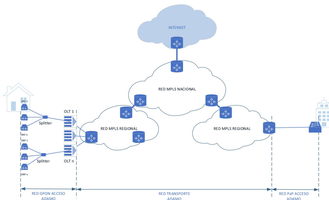
Figura 1 - Red de acceso y transporte de Adamo
